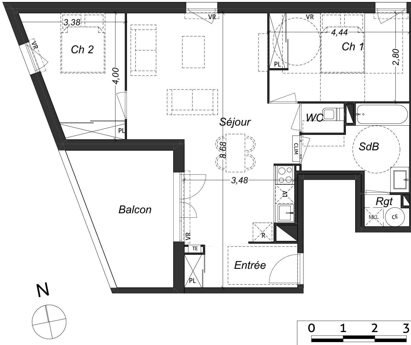
Plan de repérage R+3
